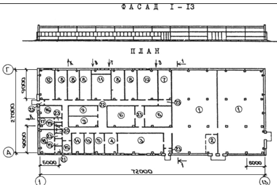
Рис.Г.5. Производственный корпус цеха по содержанию и разведению пчел-листорезов (ТП 808-5-17.86):
