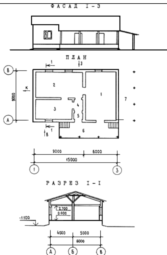
Рис.В.4. Пасечный дом для пчеловодческой фермы на 300 пчелиных семей (ТП 808-5-21.86):
