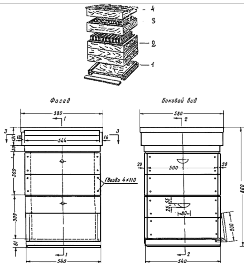
Рис.Е.1. Конструкция улья на 24 рамки:
