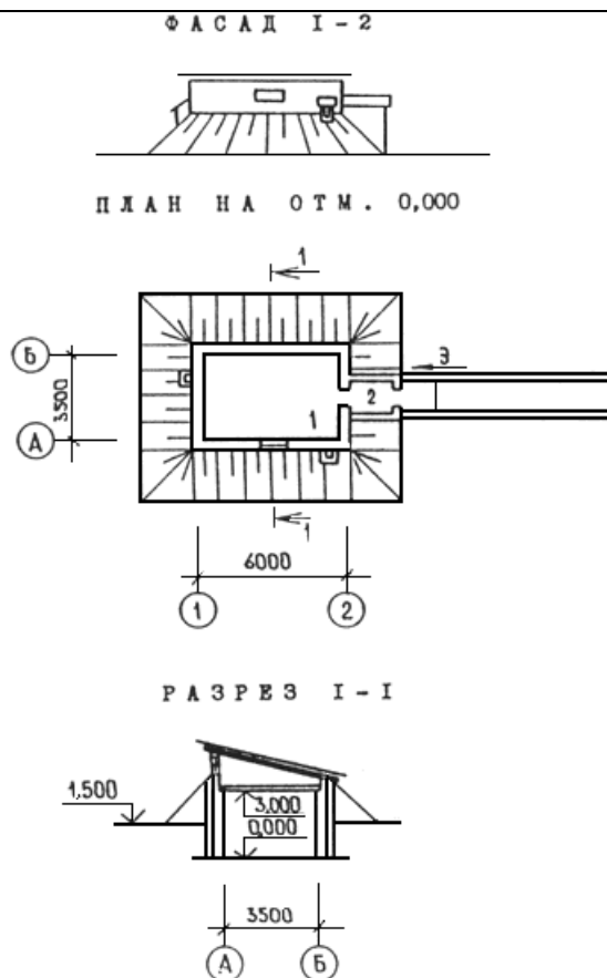
Рис.Д.1. Зимовник на 100 пчелиных семей (ТП 808-5-52.92) полузаглубленный:
