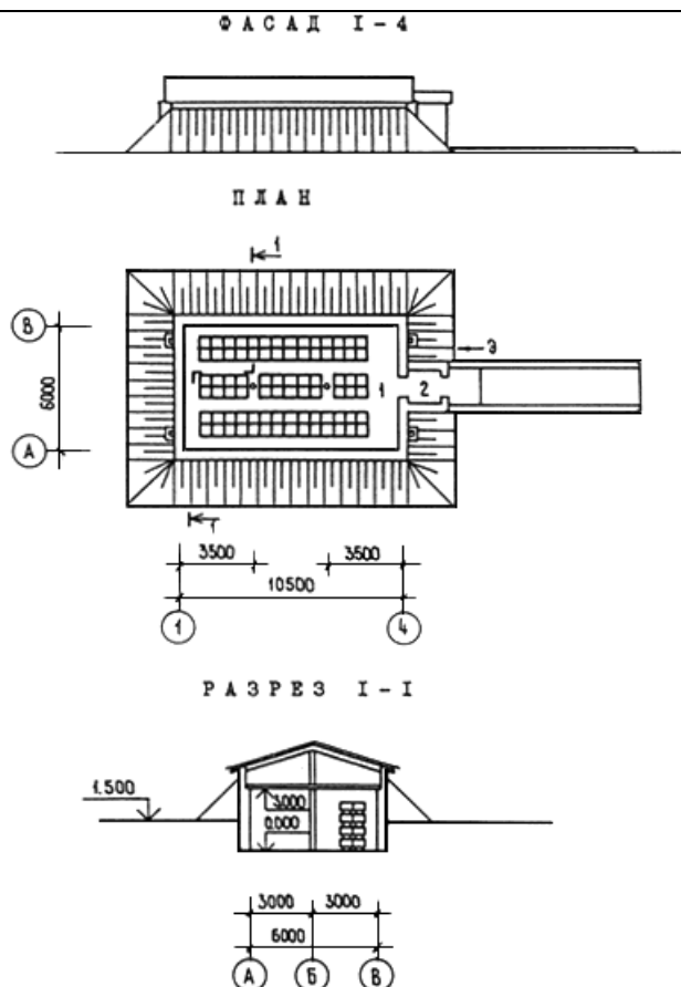
Рис.Д.7. Зимовник на 300 пчелиных семей (ТП 808-5-28.86) - полузаглубленный:
