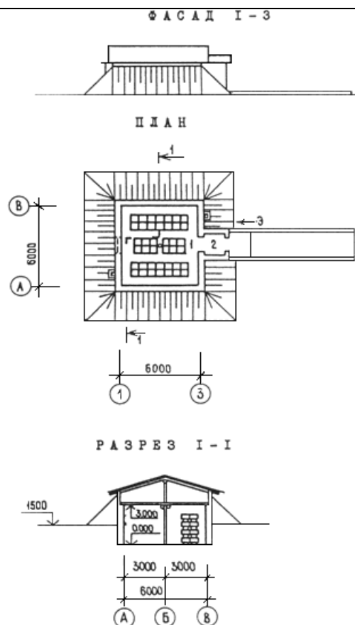
Рис.Д.2. Зимовник на 150 пчелиных семей (ТП 808-5-24.86) полузаглубленный:
