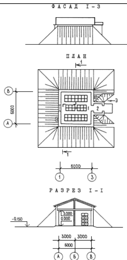
Рис.Д.3. Зимовник на 150 пчелиных семей (ТП 808-5-23.86) наземный:
