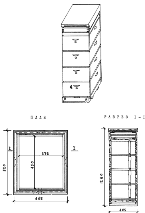
Рис.Е.7. Многокорпусный улей (ТП 808-5-1)
