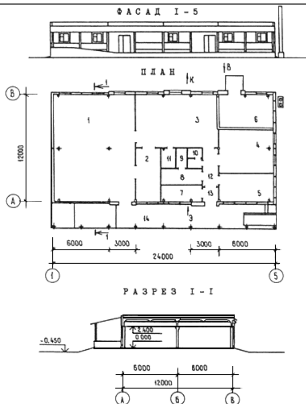
Рис.Г.1. Производственный корпус для пчеловодческой фермы на 600 пчелиных семей (ТП 808-5-40.86):
