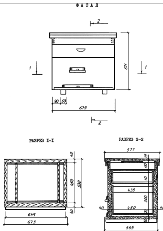
Рис.Е.3. Улей-лежак на 16 рамок с надставкой (ТП 808-5-15)
