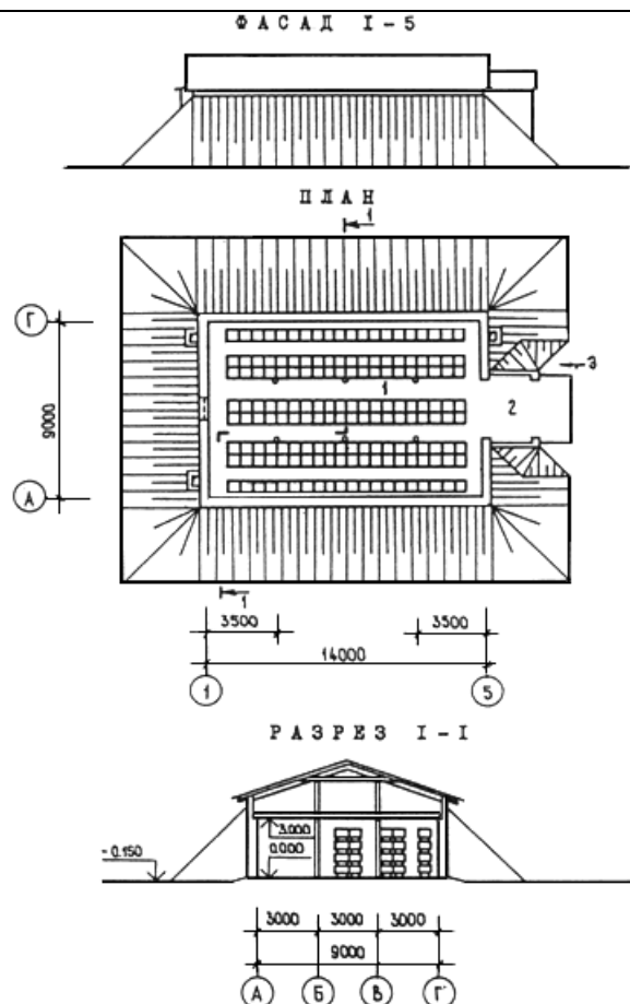
Рис.Д.9. Зимовник на 600 пчелиных семей (ТП 808-5-32.86) полузаглубленный:
