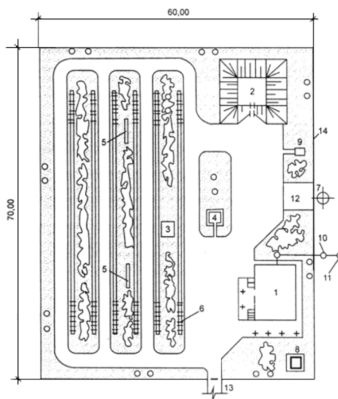
Рис.Б.1. Схема генерального плана пчеловодческой фермы на 150 пчелиных семей (ТП 808-05-18.86):
