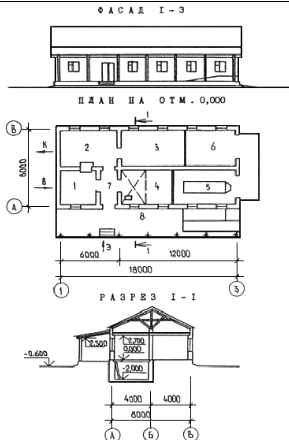
Рис.В.3. Пасечный дом с хозяйственным блоком на 200 пчелиных семей (ТП 808-5-50.92):
