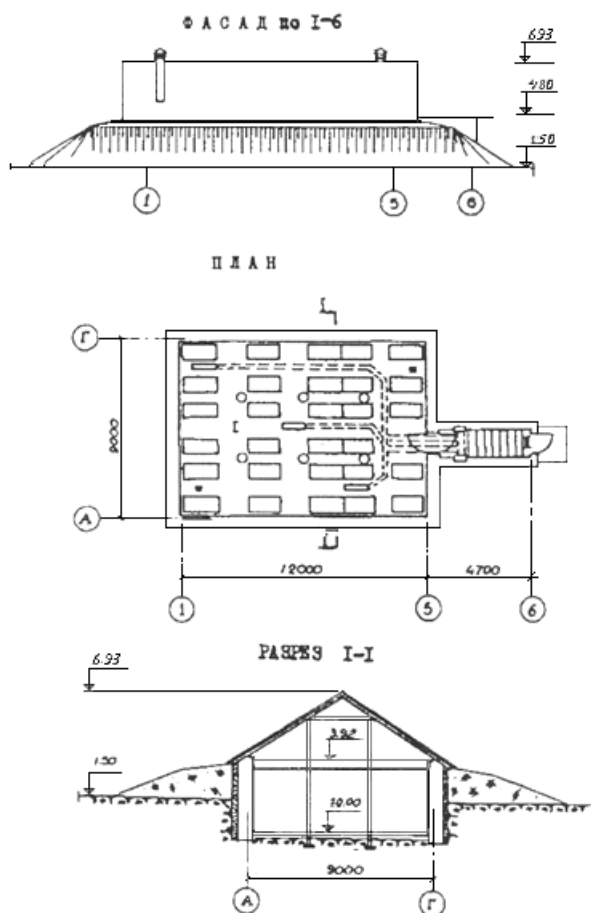
Рис.Д.5. Зимовник на 250 пчелиных семей (ТП 808-5-4) - полузаглубленный:
