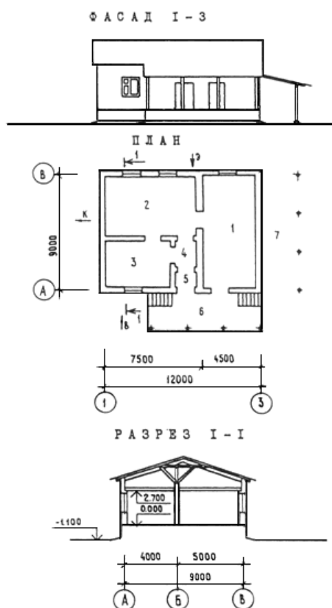
Рис.В.2. Пасечный дом для пчеловодческой фермы на 150 пчелиных семей (ТП 808-5-19.86):
