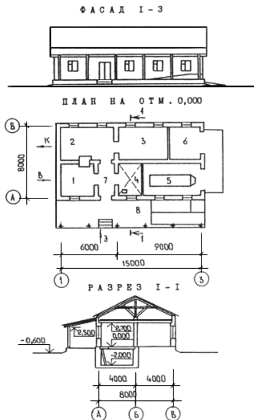
Рис.В.1. Пасечный дом с хозяйственным блоком на 100 пчелиных семей (ТП 808-5-48.92):
