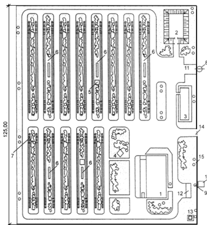
Рис.Б.3. Схема генерального плана пчеловодческой фермы на 600 пчелиных семей (ТП 808-05-18.86):
