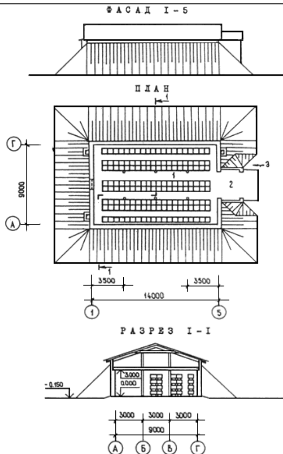
Рис.Д.8. Зимовник на 600 пчелиных семей (ТП 808-5-31.86) наземный:
