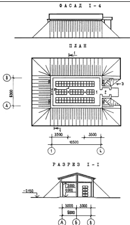
Рис.Д.6. Зимовник на 300 пчелиных семей (ТП 808-5-27.86) наземный:
