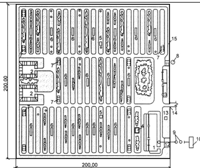
Рис.Б.5. Схема генерального плана пчеловодческой фермы на 2400 пчелиных семей (ТП 808-05-18.86):
