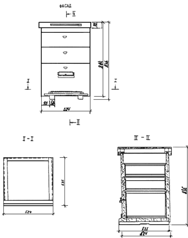
Рис.Е.5. Улей однокорпусный с двумя магазинами (ТП 808-5-14)
